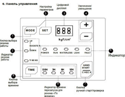
Старая версия контроллера
